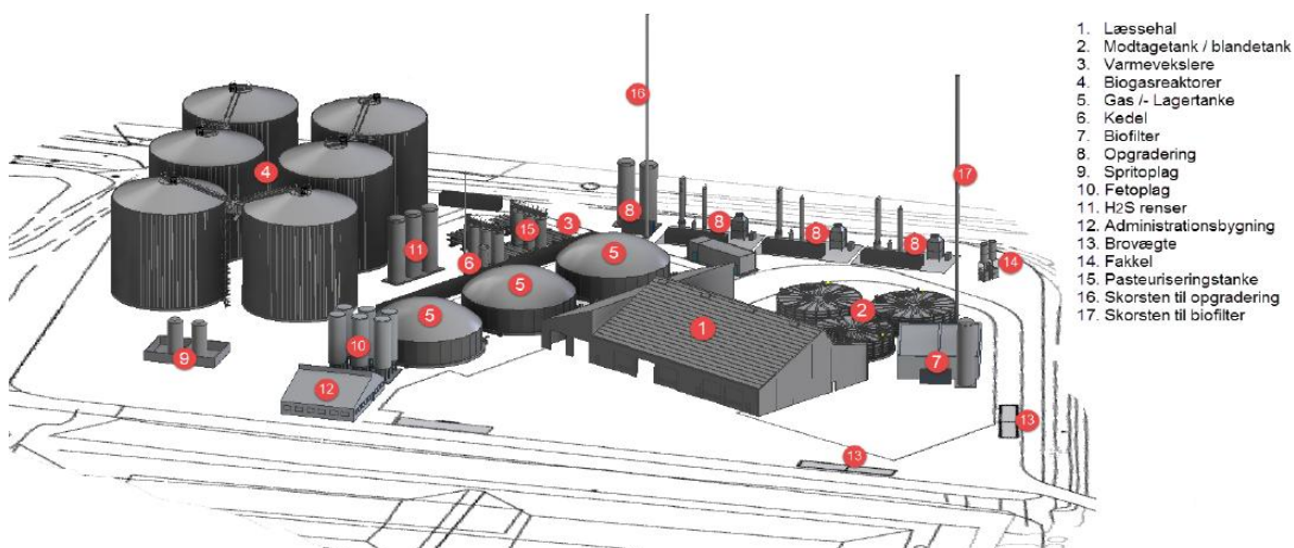
Kalundborg Bioenergi, anlægslayout.
