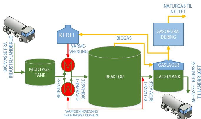
Figur 1: Principdiagram, Kalundborg Bioenergi
